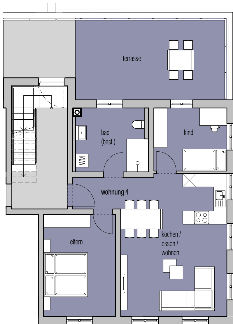
obergeschoss wohnung 4
